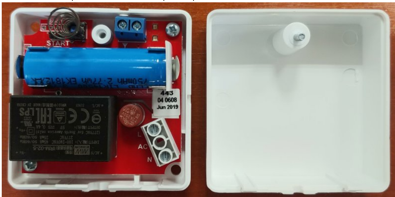
Рисунок 1. Ретранслятор с открытой крышкой
